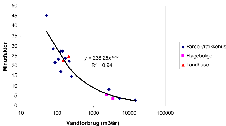
Figur 4.1.3. Husholdningsforbrug. Minutfaktorer som funktion af vandforbruget.
