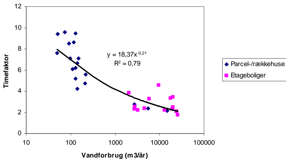
Figur 4.1.2. Husholdningsforbrug. Timefaktorer som funktion af vandforbruget.
